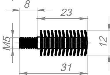
Основные размеры резьбовой вставки
