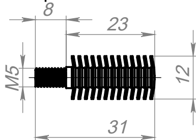
Основные размеры резьбовой вставки
