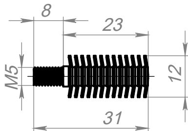
Основные размеры резьбовой вставки
