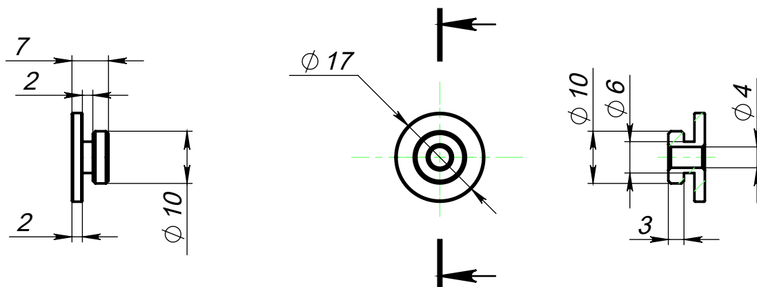
Внешний вид ADV W043
