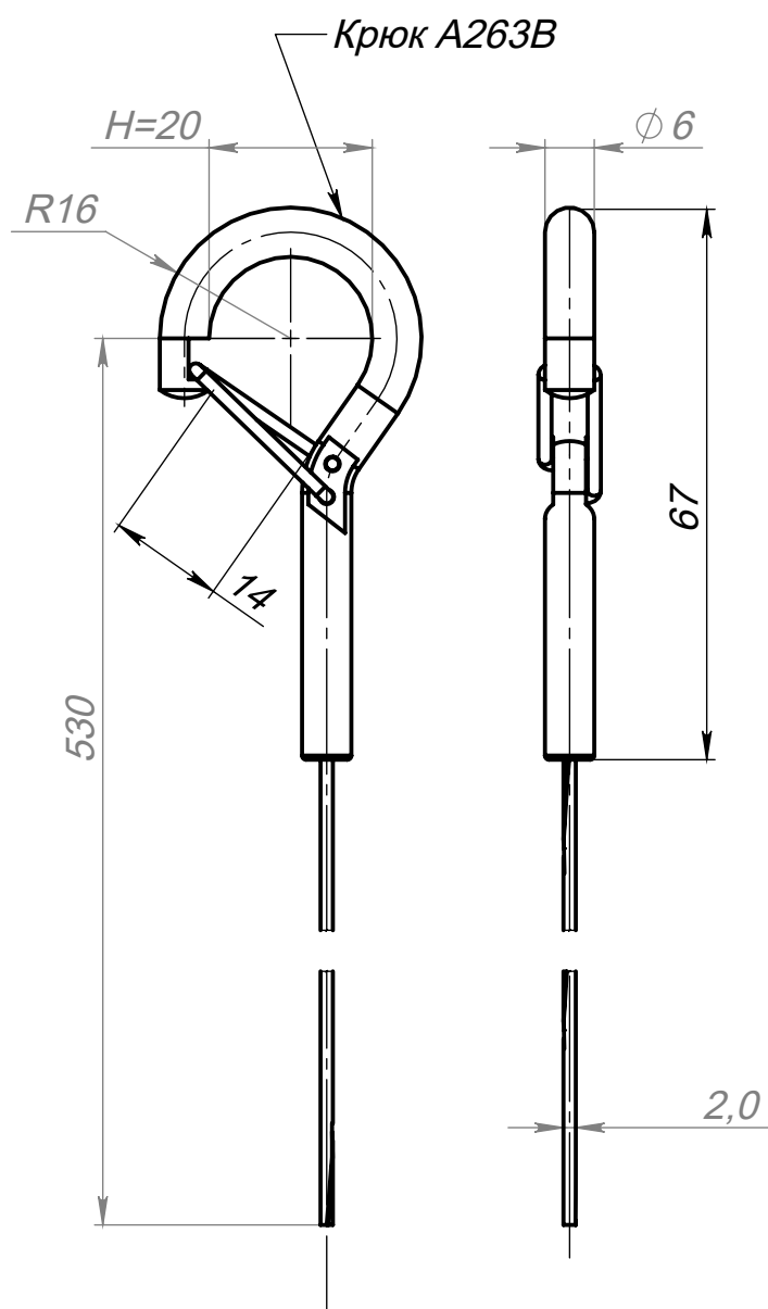
Тип наконечника Крюк А 263 В
