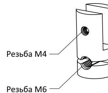
Вид без винтов зажима:
