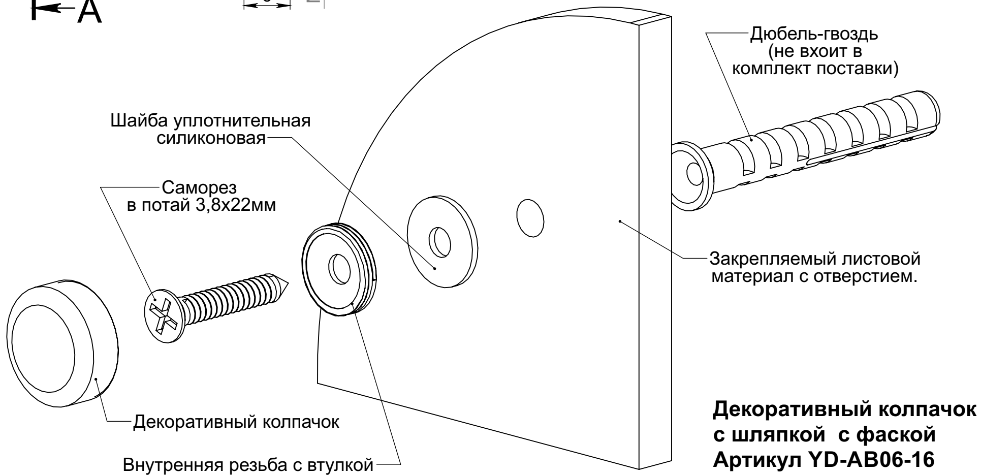
Схема применения:
